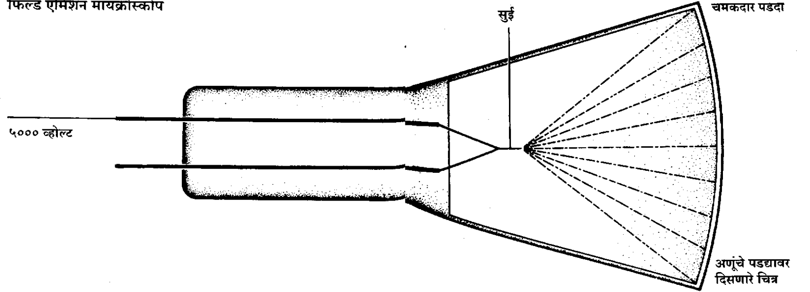
फिल्ड एमिशन मायक्रोस्कोप
