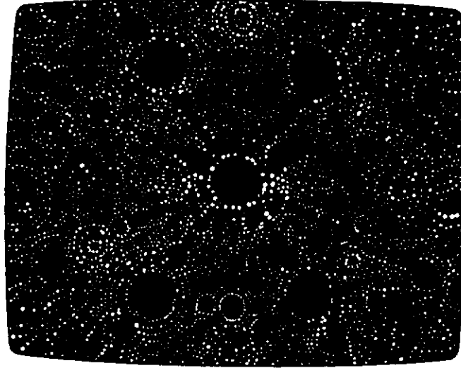
टंगस्टेनच्या स्फटिकातील अणू फिल्ड एमिशन मायक्रोस्कोपच्या पडद्यावर ठिपक्यासारखे दिसतात.
